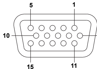
D-Sub 15-pin receptacle
